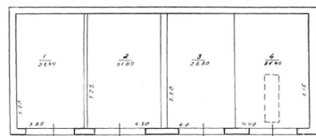
Потажный план - нежилое здание (1 этаж)
