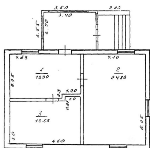
Потажный план - нежилое здание - стандартный дом (1 этаж)
